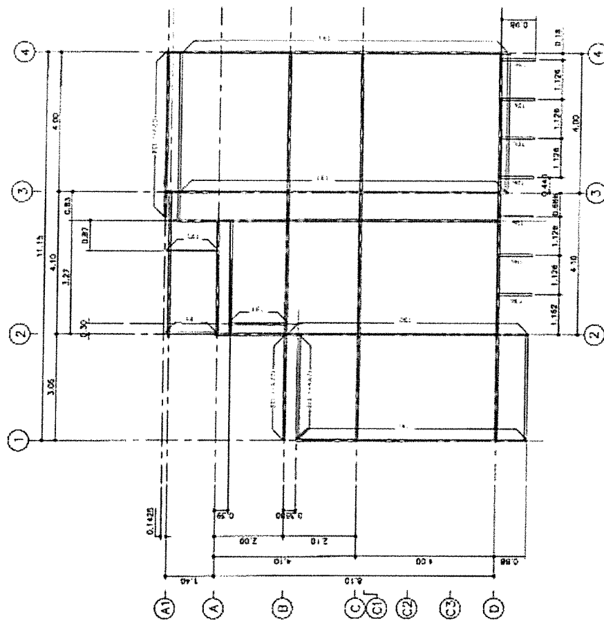
แปลนโครงสร้างชั้นกัน
