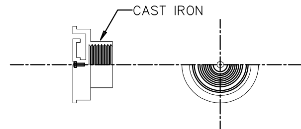
แบบขยายฝาปิดท่อระบายอากาศชนิดด้านข้าง (AVC.)
