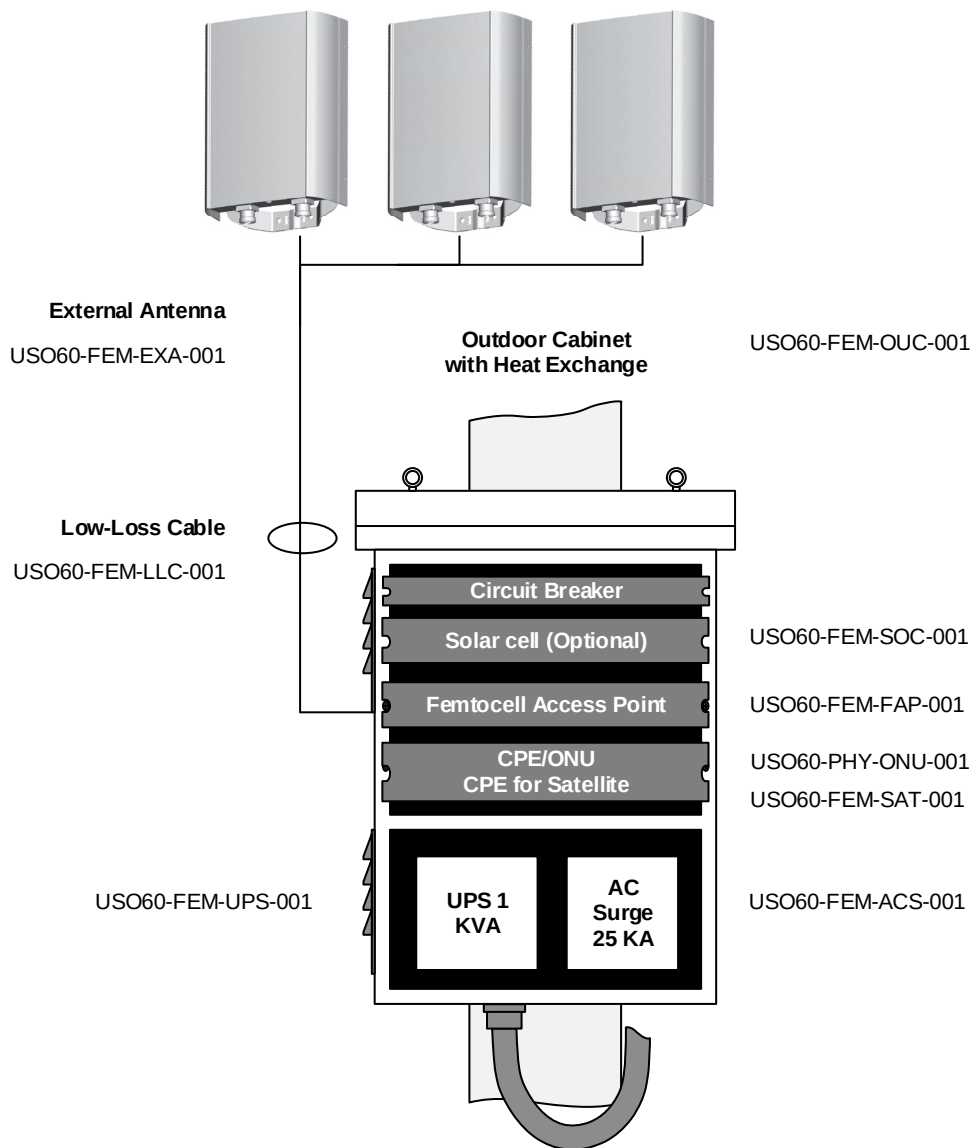
ภาพที่ 4 รายการอุปกรณ์ชุดตู้ Cellular Station: CS
